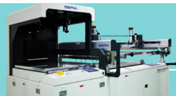
CCD カメラ付半自動印刷機
